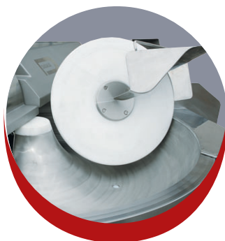
Vide cuve à manœuvre et moteur hydraulique
